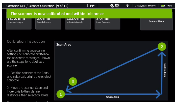
Пошаговая калибровка
